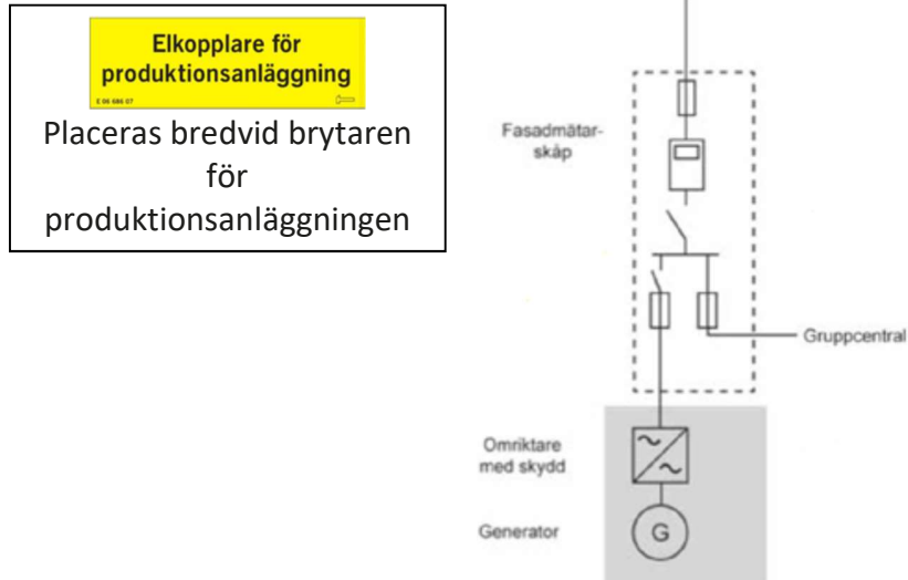
Figur 4 Exempel på märkning vid direktanslutning i mätarskåp.
